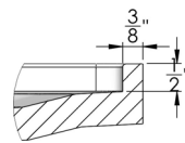
Edge Detail
