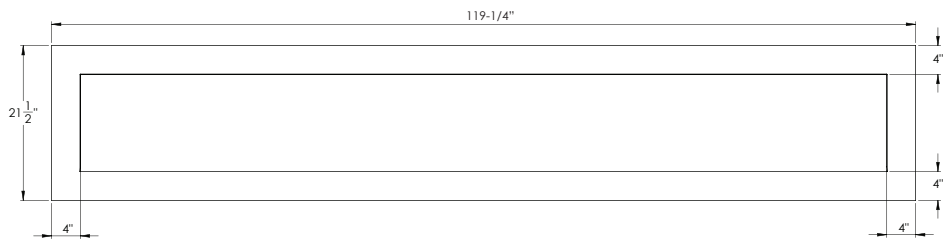
SLV04-A/B-L00R00
